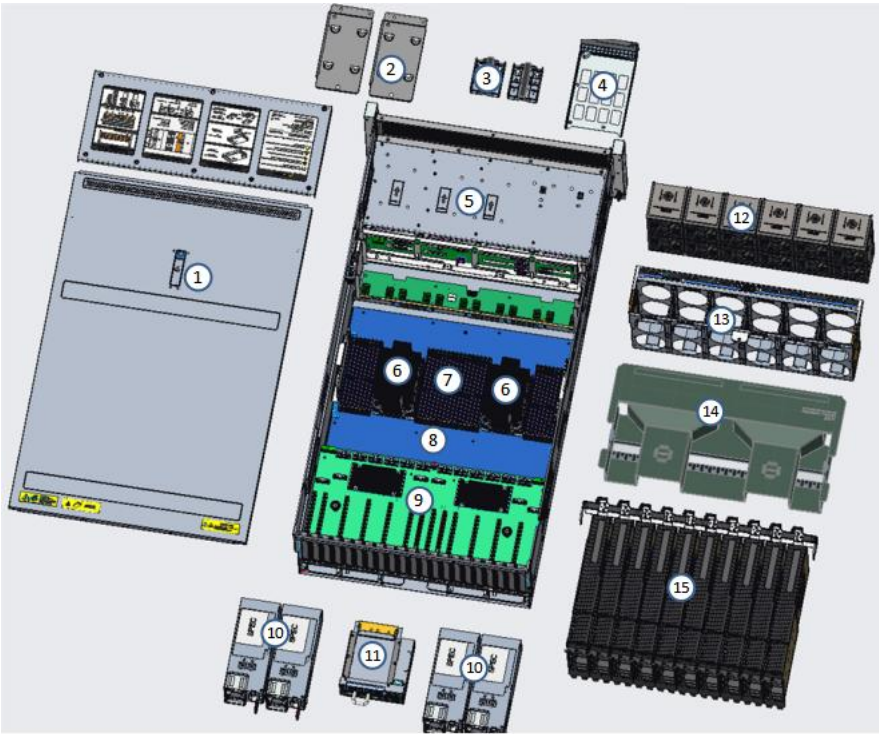
结构图 1-3
