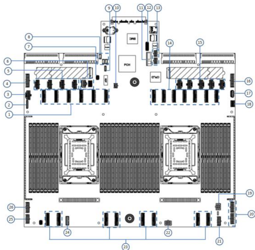
主板图 2-16
