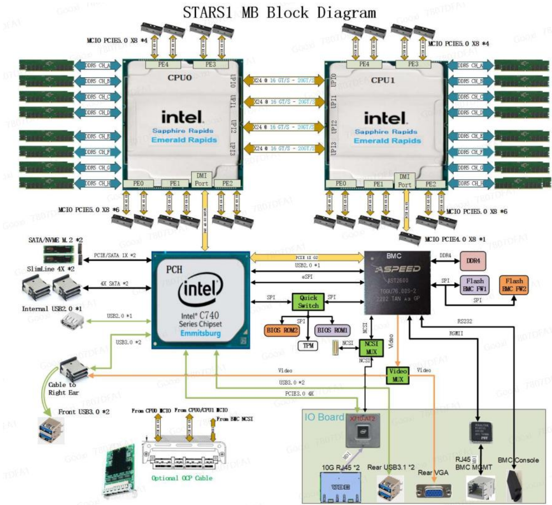
主板逻辑框图 1-4
